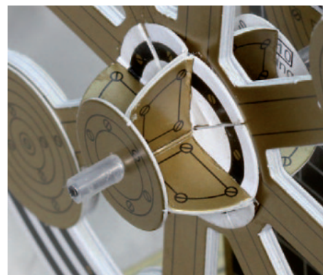
Abb. 7: Schwungradnabe
