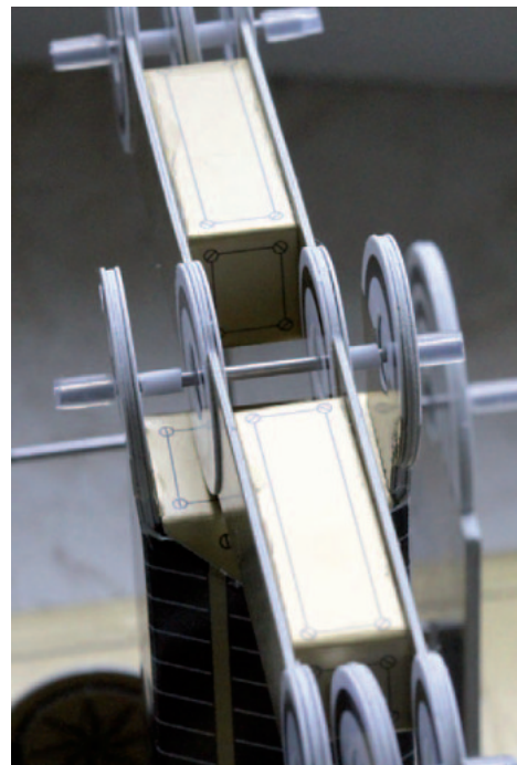
Abb. 2: Achsmontage Säule und Balancier
